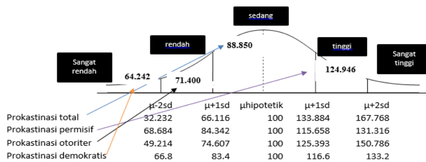
Gambar 1 grafik prokrastinasi
